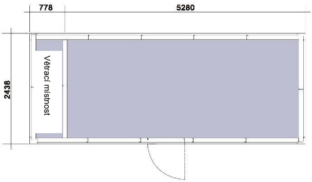
Nákres chladícího kontejnerového domu
