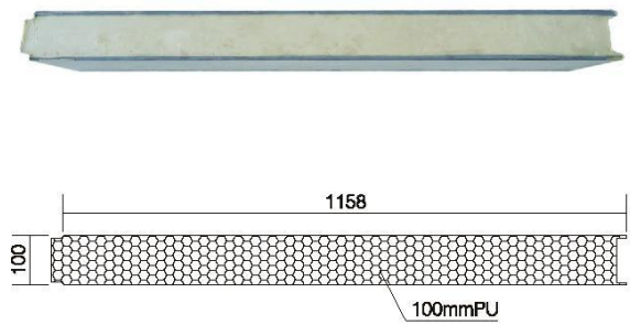
100mm PU Wall Panel, PU Density 40kg/m³, Dvojitý 0,42mm barvený ocelový povrch
